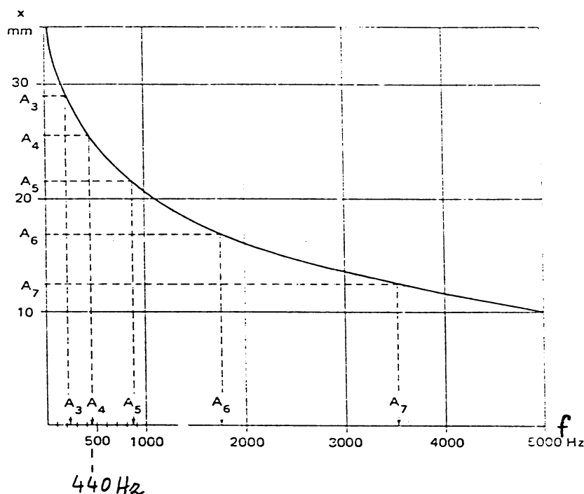
Figura 2.7: Posizione della zona di risonanza sulla membrana basilare
