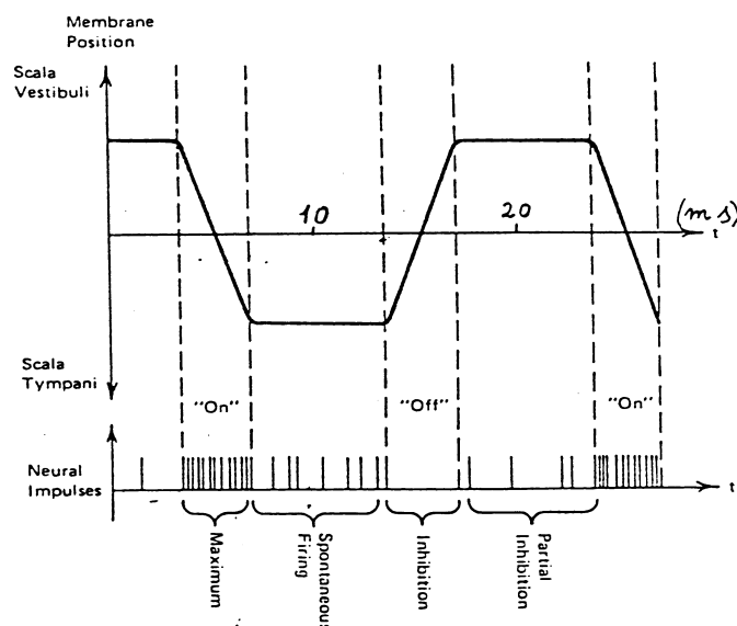
Figura 2.20: Treno di impulsi generato da un'onda periodica
