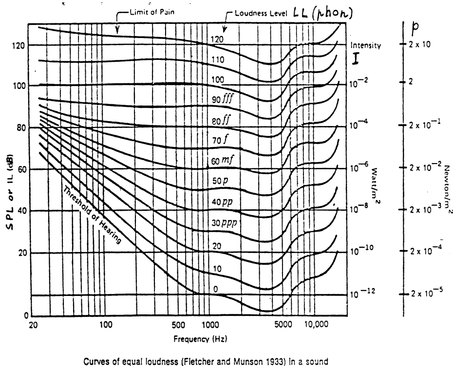
Figura 2.25: Curve di eguale intensità percepita (Fletcher and Munson, 1933)
