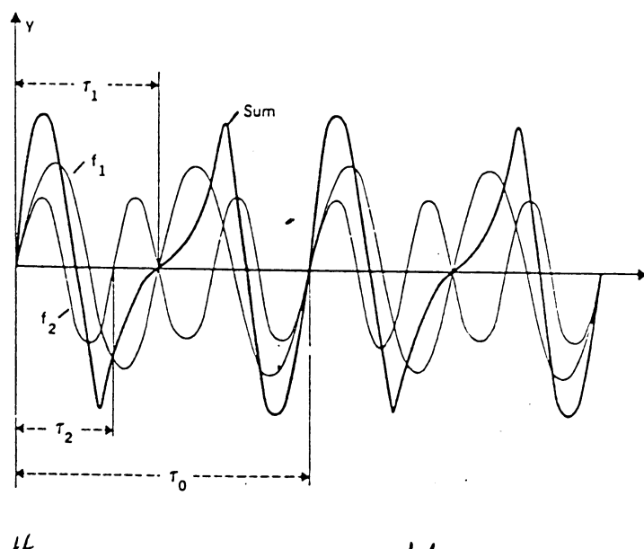
Figura 2.18: Ricostruzione della fondamentale ( \tau_1 = \frac{1}{f_1} , \tau_2 = \frac{1}{f_2} , \tau_0 = \frac{1}{f_0} )
