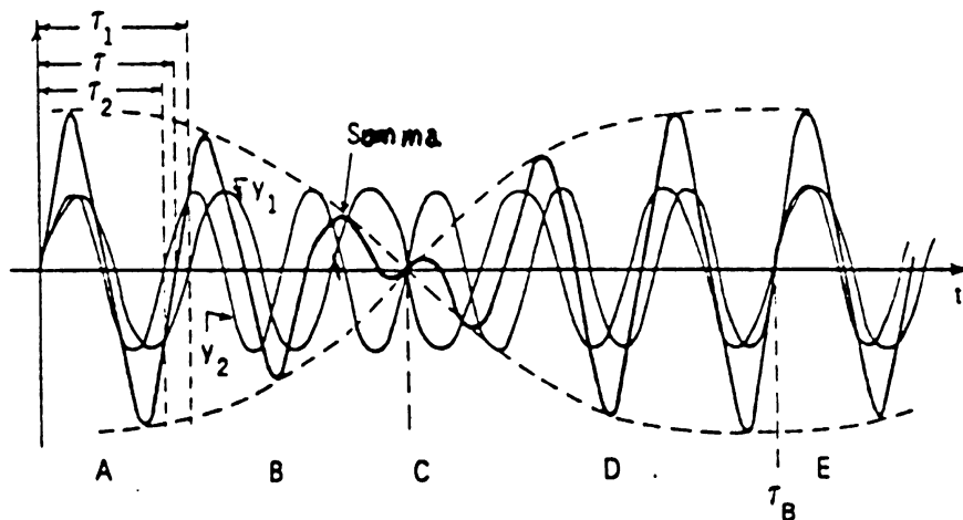
Figura 2.13: Battimenti del I ordine: pitch risultante ( \tau_1 = \frac{1}{f_1} , \tau_2 = \frac{1}{f_2} , \tau = \frac{1}{f} )
