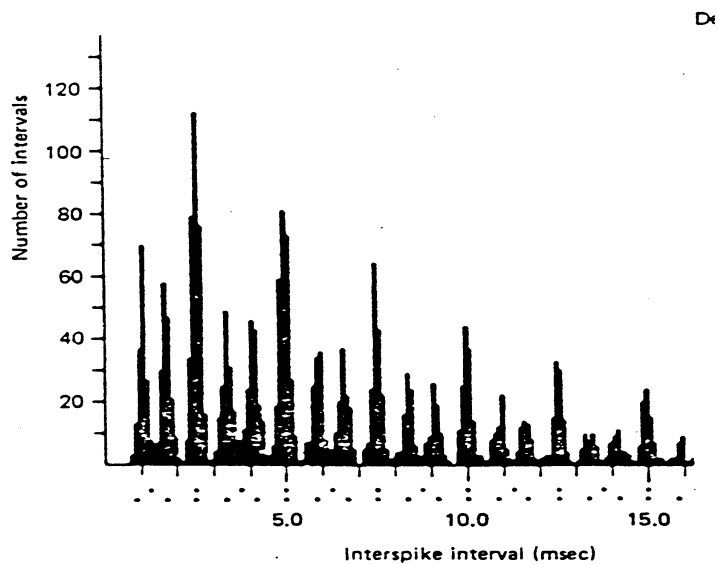
Figura 2.21: Istogramma del numero di occorrenze di dato tempo di intercorrenza fra spike successivi nel nervo uditivo a fronte di un eccitazione composta da due suoni puri
