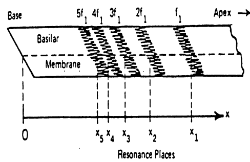
Figura 2.23: Pattern spaziale sulla membrana basilare dovuto a un suono armonici
