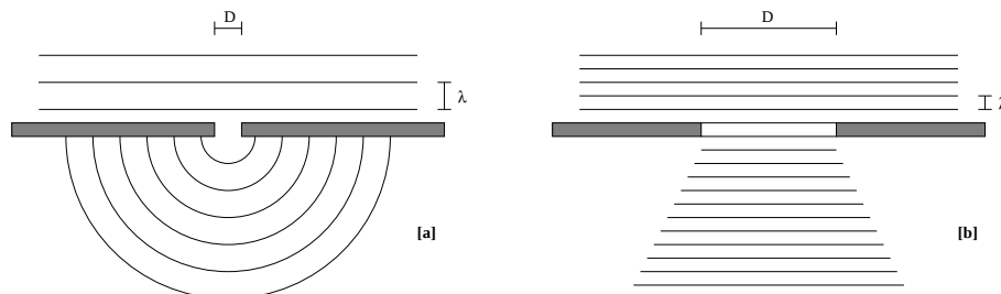
Figura 2.3: Effetto della diffrazione nei casi \lambda > D in [a] e \lambda < D in [b]
