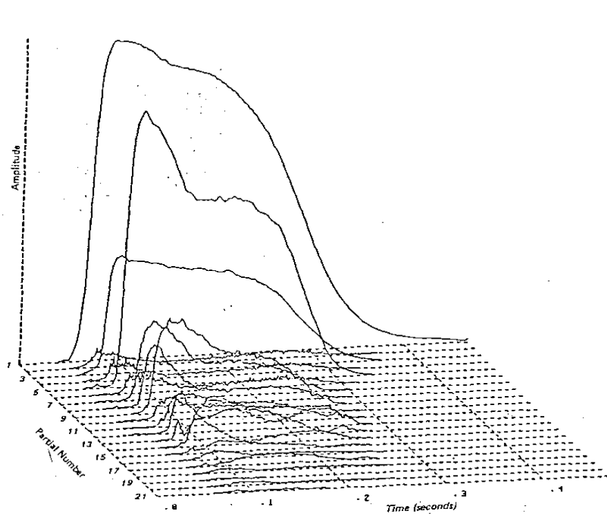
Figura 2.30: Rappresentazione tempo-frequenza di un suono
