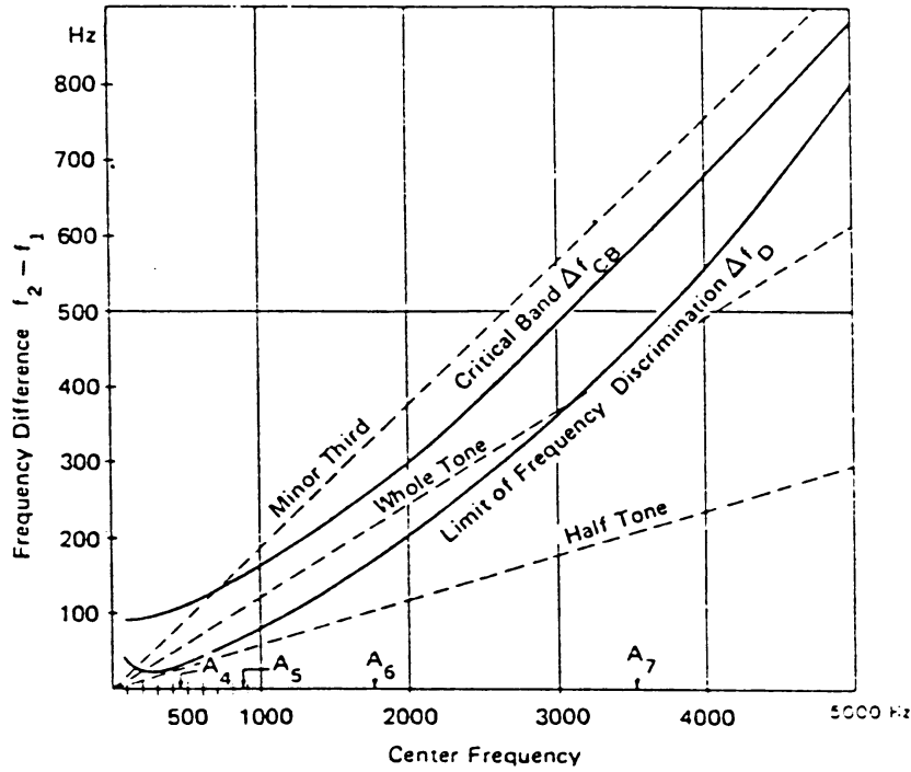
Figura 2.15: Banda critica e discriminazione del pitch al variare della frequenza centrale
