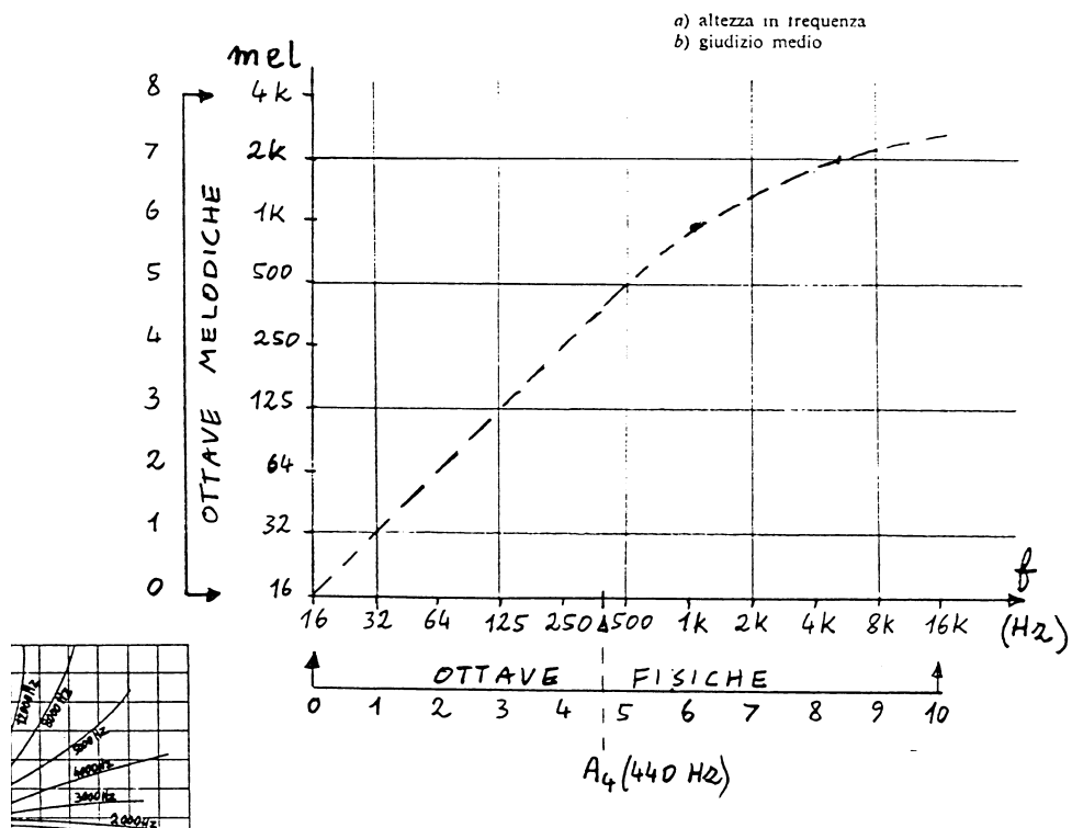
Figura 2.9: Scala mel
