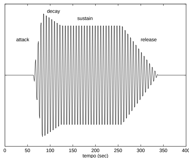
Figura 2.2: Evoluzione del segnale musicale nel tempo: sono evidenziate le parti di attack , decay , sustain e release
