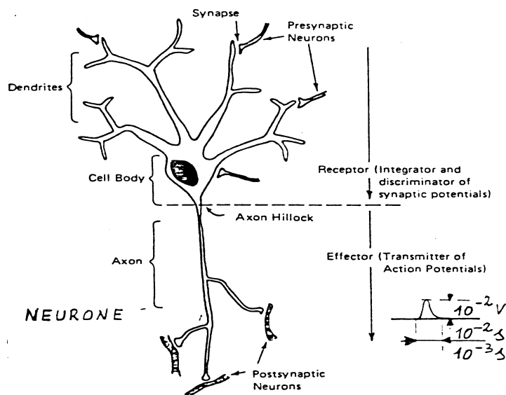
Figura 2.19: Neurone
