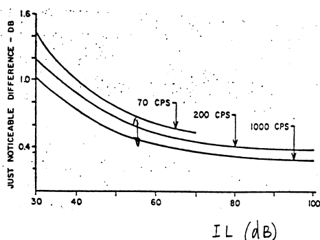
Figura 2.24: Valori di jnd di intensità per valori diversi di IL e frequenza del suono puro
