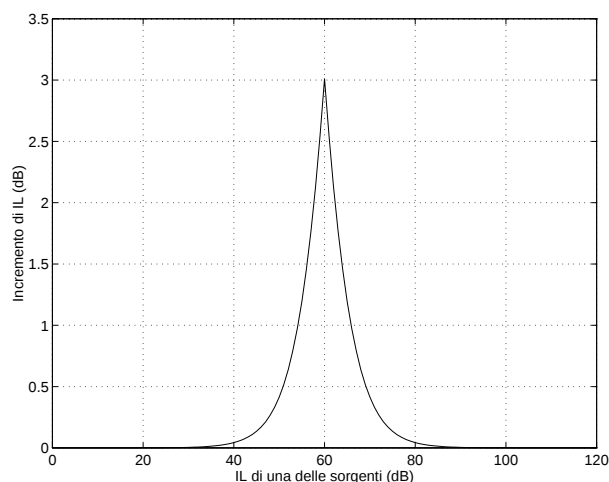
Figura 2.4: Incremento del livello di intensità nel caso di due sorgenti, la prima fissa a 60 dB e la seconda variabile da 0 dB a 120 dB
