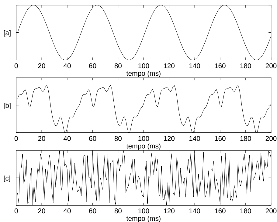
Figura 2.1: Andamento nel tempo di tre segnali rispettivamente con andamento: [a] sinusoidale, [b] periodico (somma di 15 sinusoidi), [c] aperiodico
